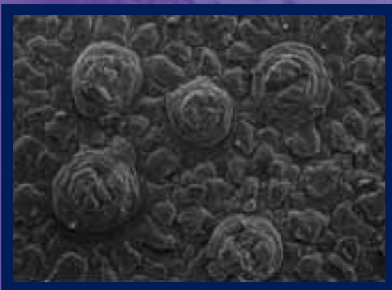
DEHP 5 Jahre, 40-fach vergrößert Freibewitterung Nordsee (Sylt)
