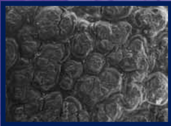
DEHP 2 Jahre, 40-fach vergrößert Freibewitterung Nordsee (Sylt)
