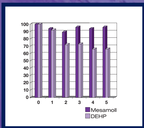
Veränderung der Bruchdehnung nach Bewitterung im Nordseeklima
