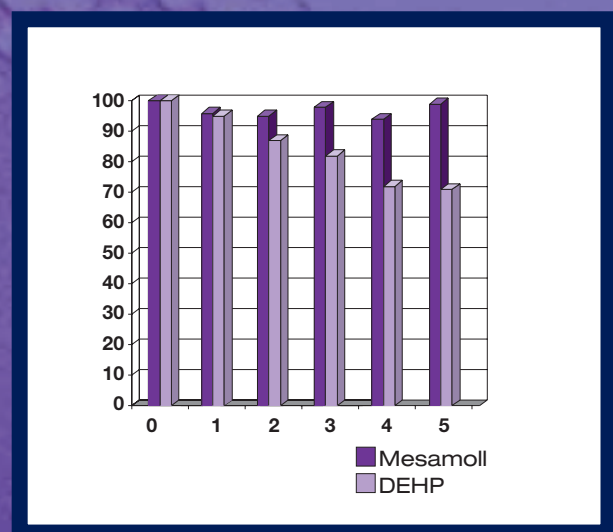
Veränderung der Zugfestigkeit nach Bewitterung im Nordseeklima
